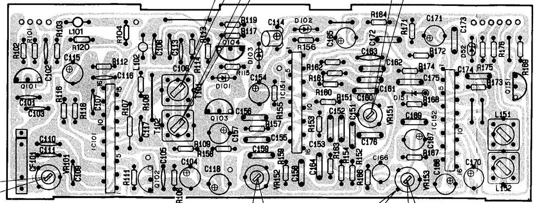
PCB-5 IF MPX P.C. Board
